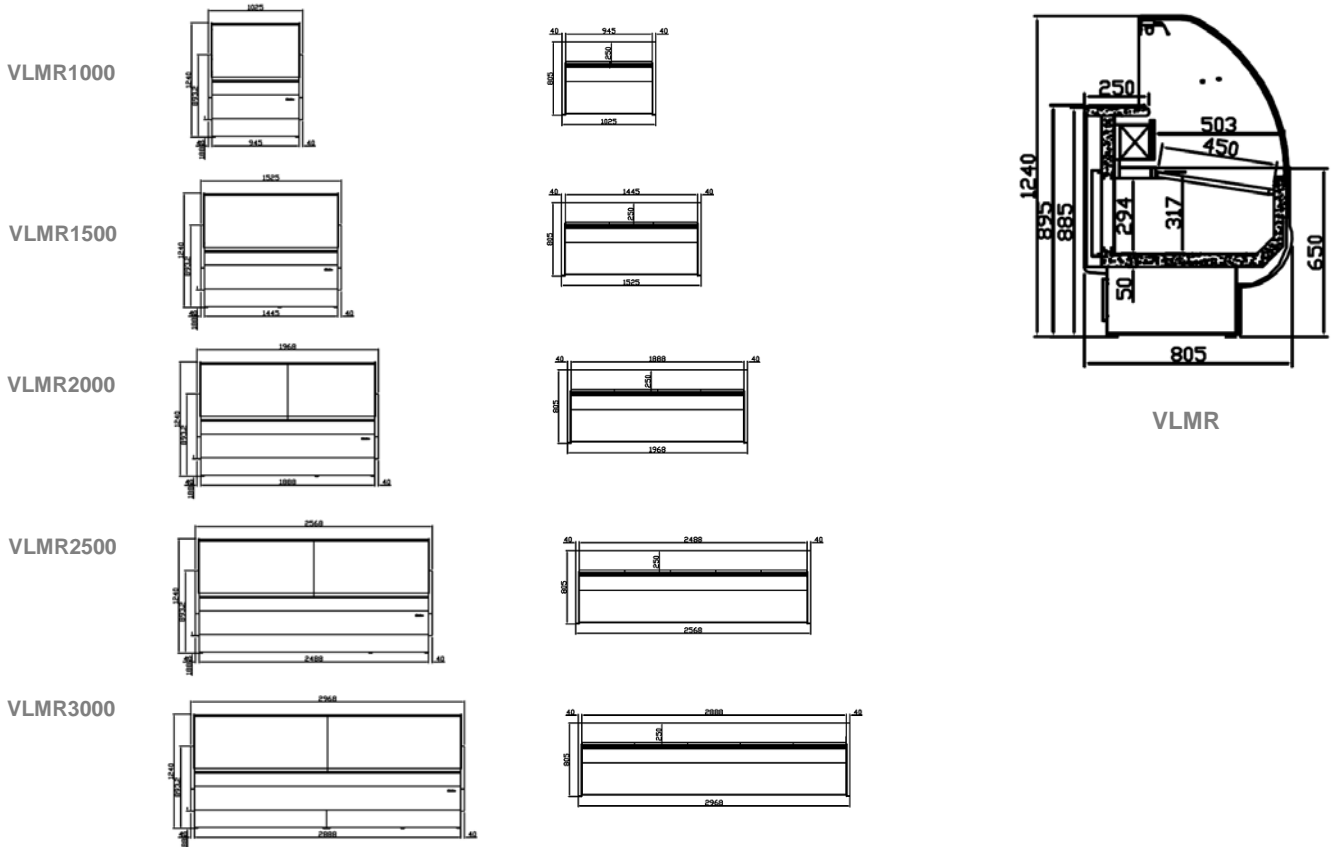
ALZADO
